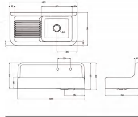
NH-8004-R L 1070 x W 530 x H 410MM
