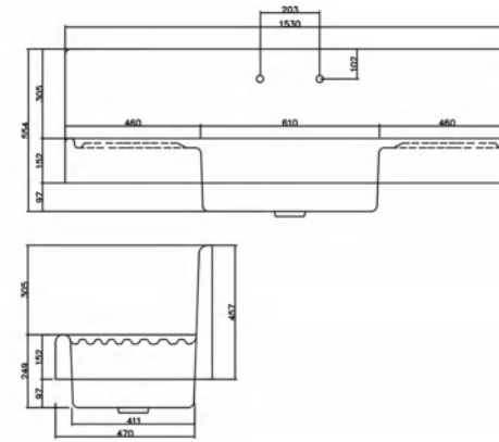
NH-8005 L 1530 x W 470 x H 554MM
