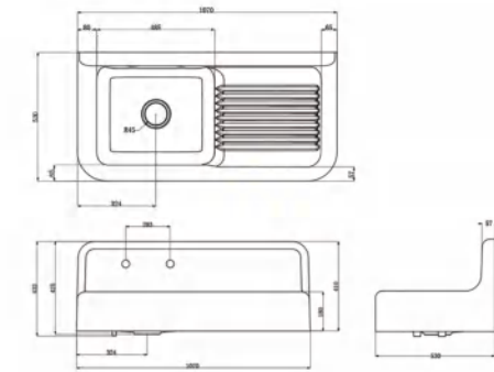
NH-8004-R L 1070 x W 530 x H 410MM
