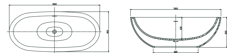
Milano-1800 型号: PB1031 尺寸: 1800x800x600mm
